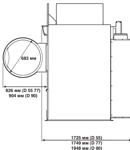
ВИД СБОКУ D 55 77 90
